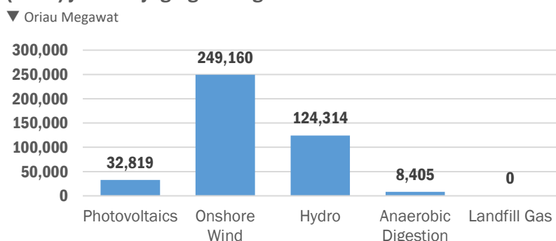
Ffigur 7.37: Trydan Adnewyddadwy a Gynhyrchwyd (MWh) yn 2020 yng Ngheredigion
