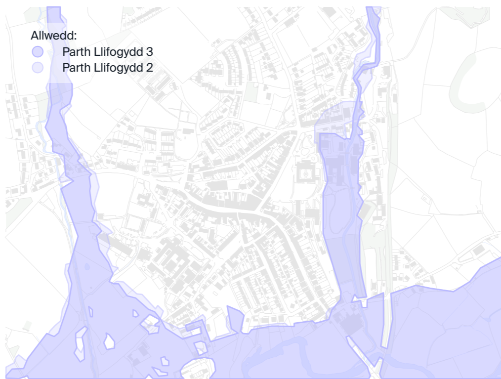
Parthau llifogydd gyda'r Map Llifogydd ar gyfer Cynllunio (FMfP)
