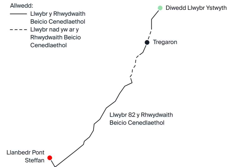
Llwybr 20 km o ddiwedd Llwybr Ystwyth i Lanbedr Pont Steffan
