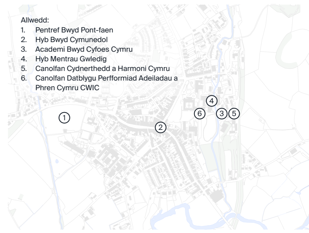
Cynigion o ran Tir Glas a safleoedd posibl
