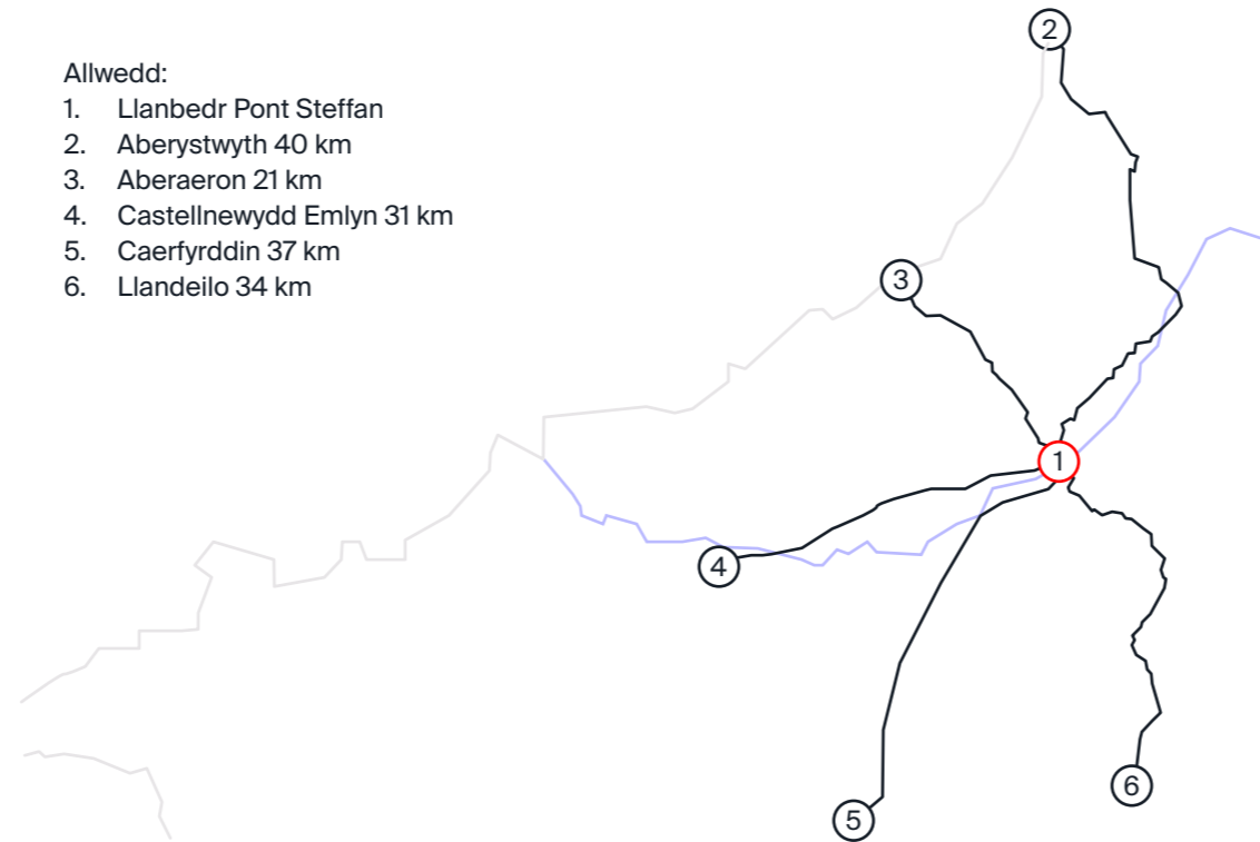
Strategaeth Adfywio Llanbedr Pont Steffan
