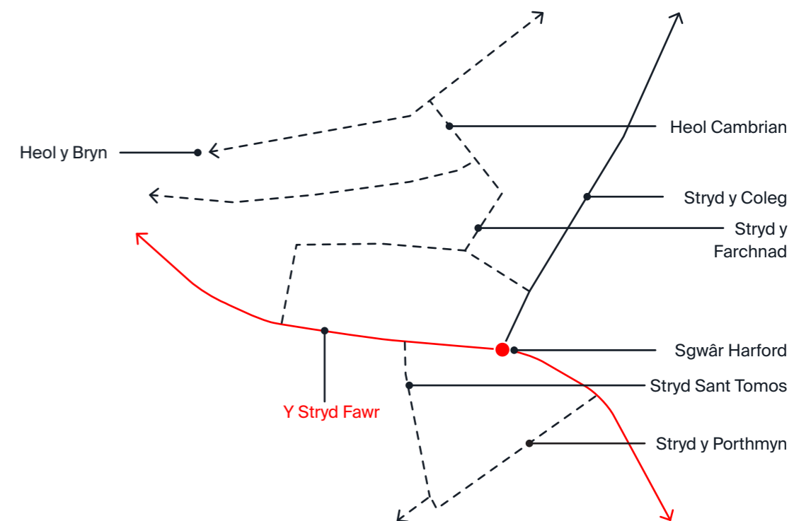
Y berthynas rhwng y Stryd Fawr a'r strydoedd cefn
