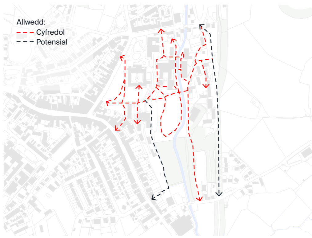
Mynediad cyfredol a phosibl i gerddwyr i'r brifysgol
