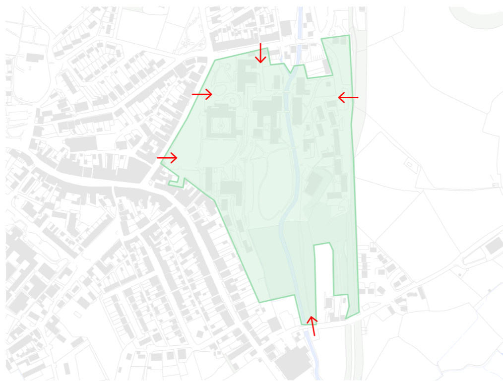
Mynedfeydd cyfredol i'r brifysgol
