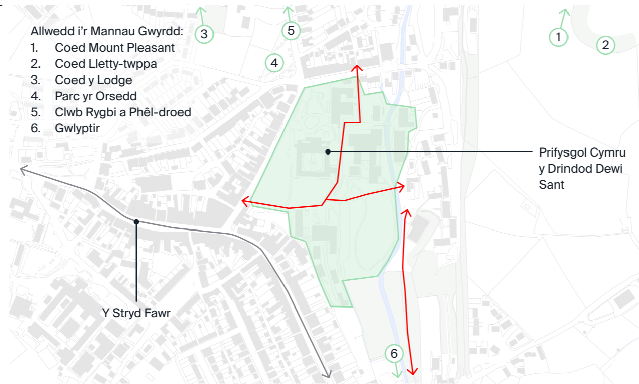
Llanbedr Pont Steffan: y cyswllt prifysgol
