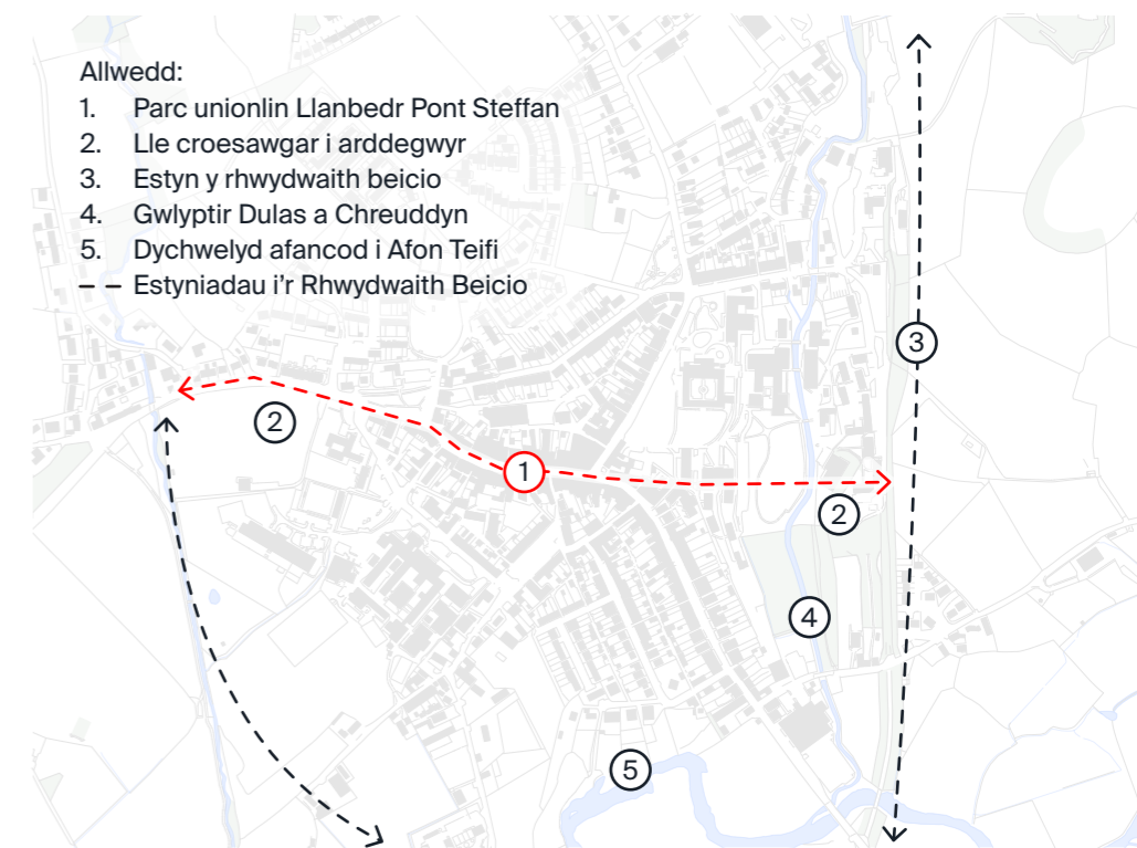
Cysylltu cyfleoedd ar gyfer seilwaith gwyrdd a glas ledled y dref
